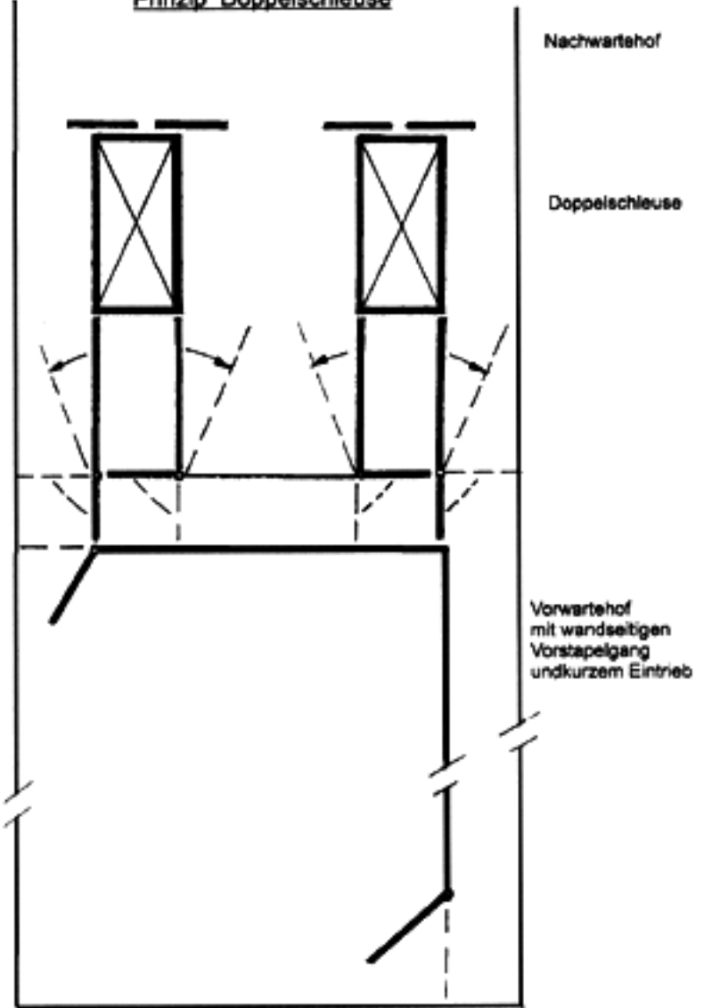
Prinzip Doppelschleuse
